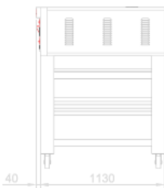
VISTA LATERALE + SUPPORTO SIDE VIEW + STAND
